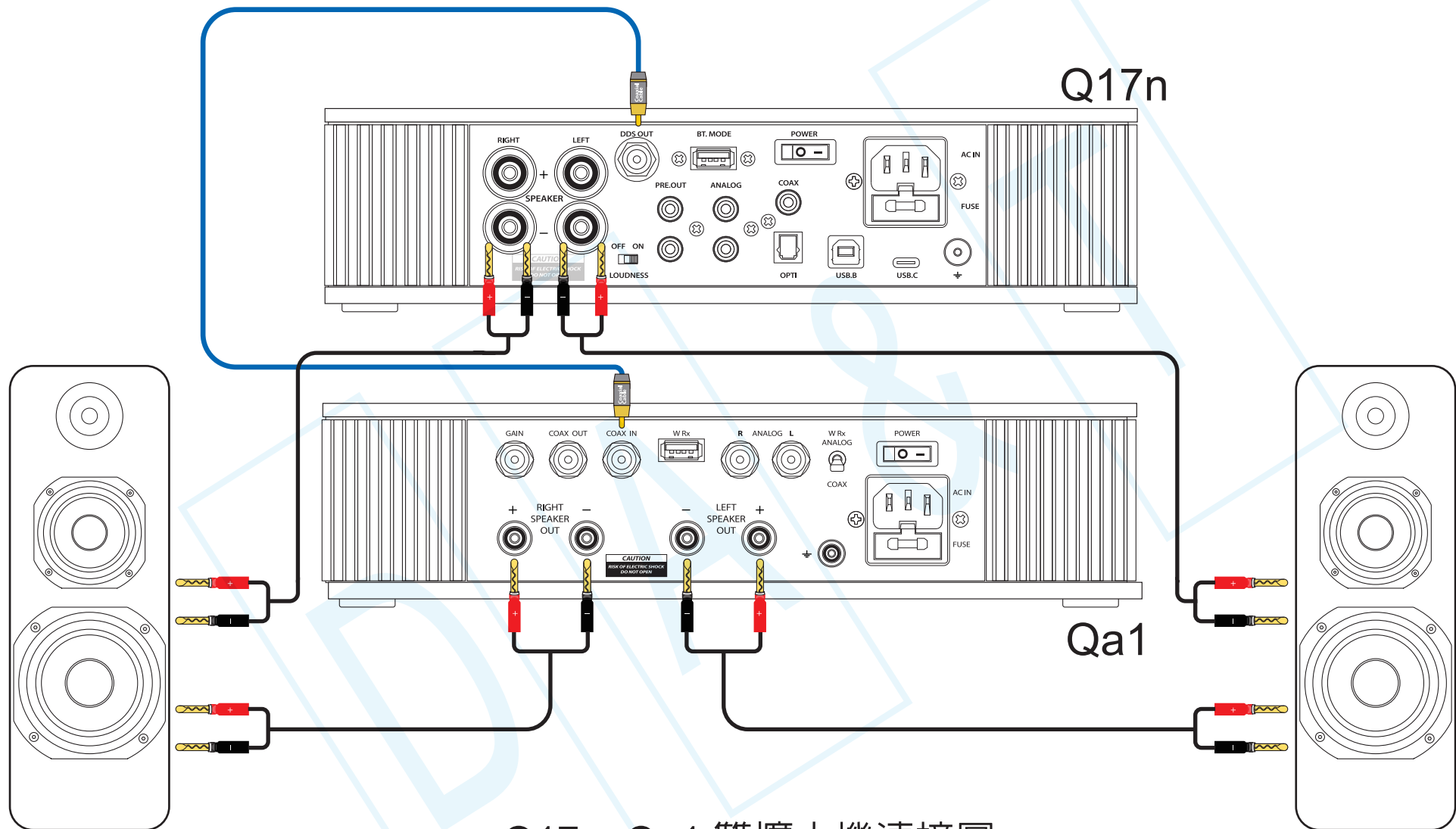
Q17n+Qa1 雙擴大機連接圖
