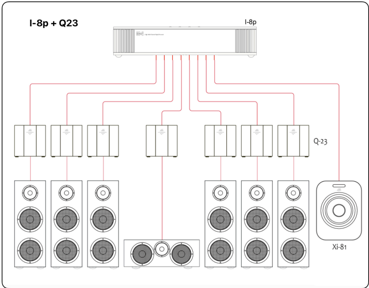
圖六：i-8p + Q23
